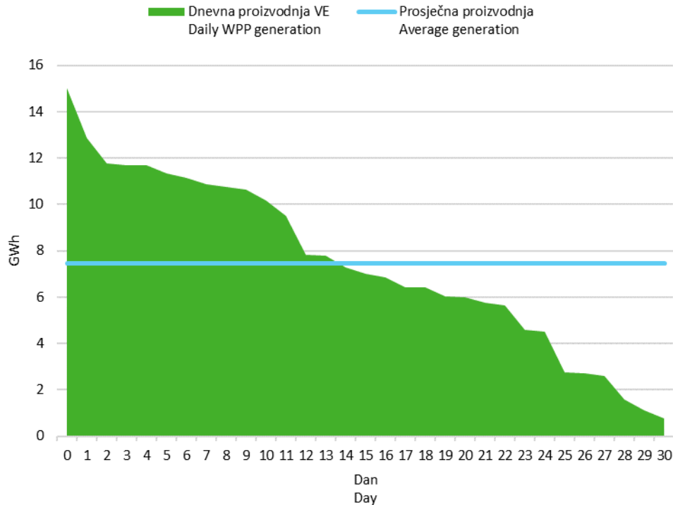
Slika 6 Krivulja trajanja dnevne proizvodnje vjetroelektrana u siječnju 2021. godine
