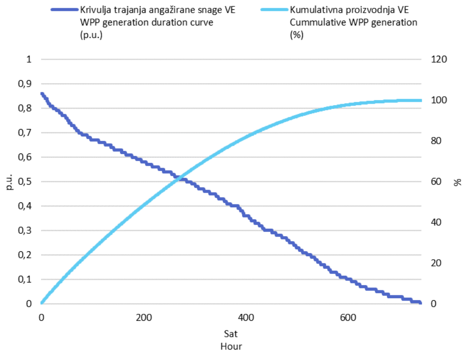
Slika 3 Krivulja trajanja angažirane snage svih VE i kumulativna proizvodnja VE u siječnju 2021. godine u jediničnim vrijednostima
