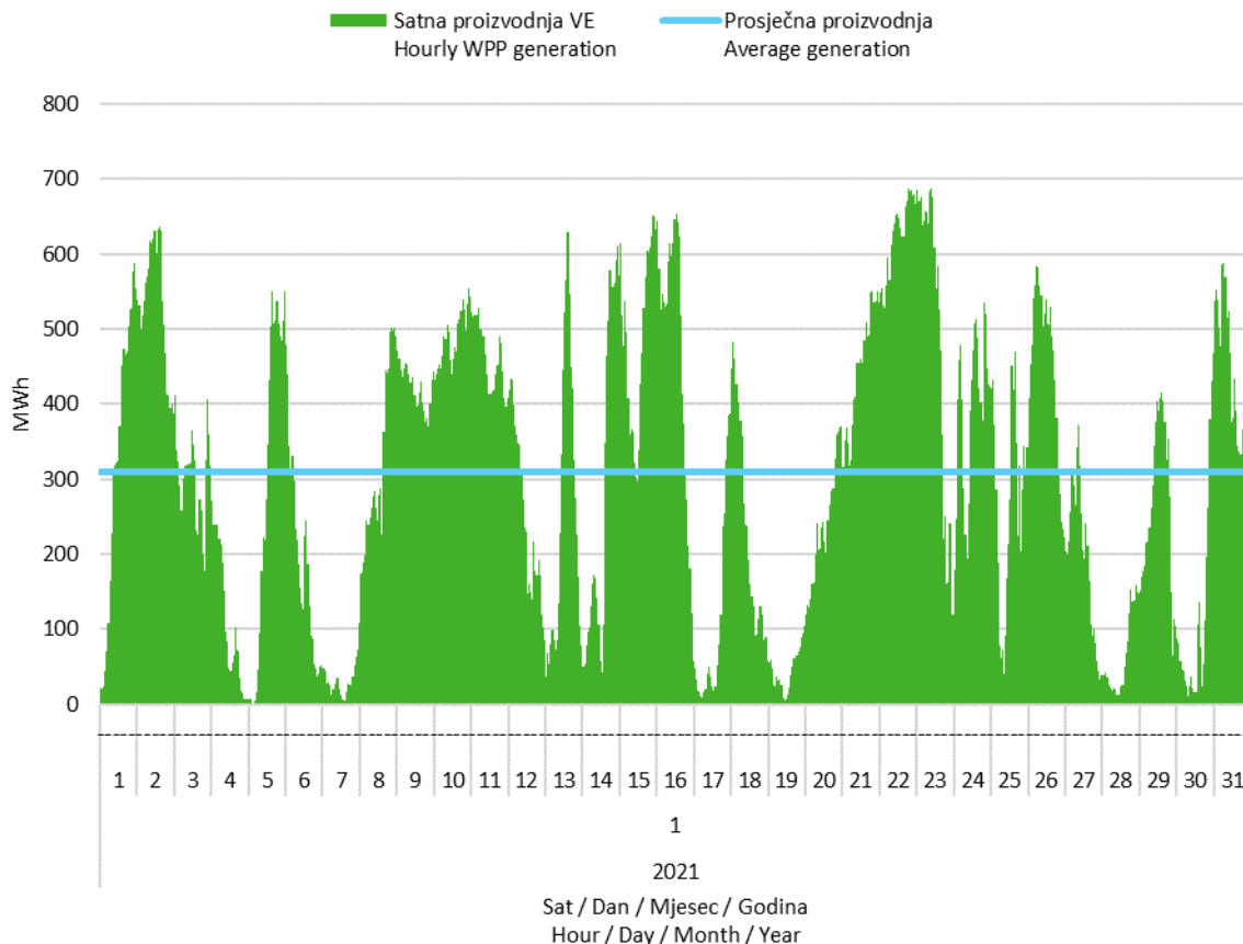
Slika 2 Satna proizvodnja svih vjetroelektrana u siječnju 2021. godine
