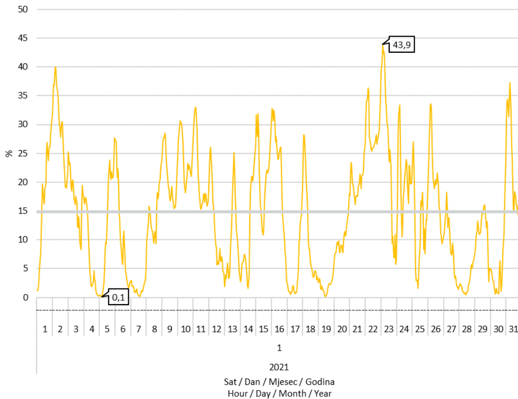
Slika 8 Udio proizvodnje vjetroelektrana u pokrivanju satnog opterećenja elektroenergetskog sustava u siječnju 2021. godine
