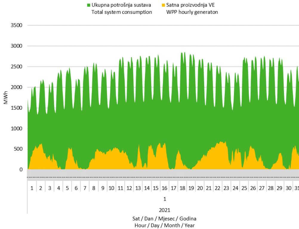
Slika 7 Usporedba satnog dijagrama opterećenja sustava i proizvodnje vjetroelektrana u siječnju 2021. godine
