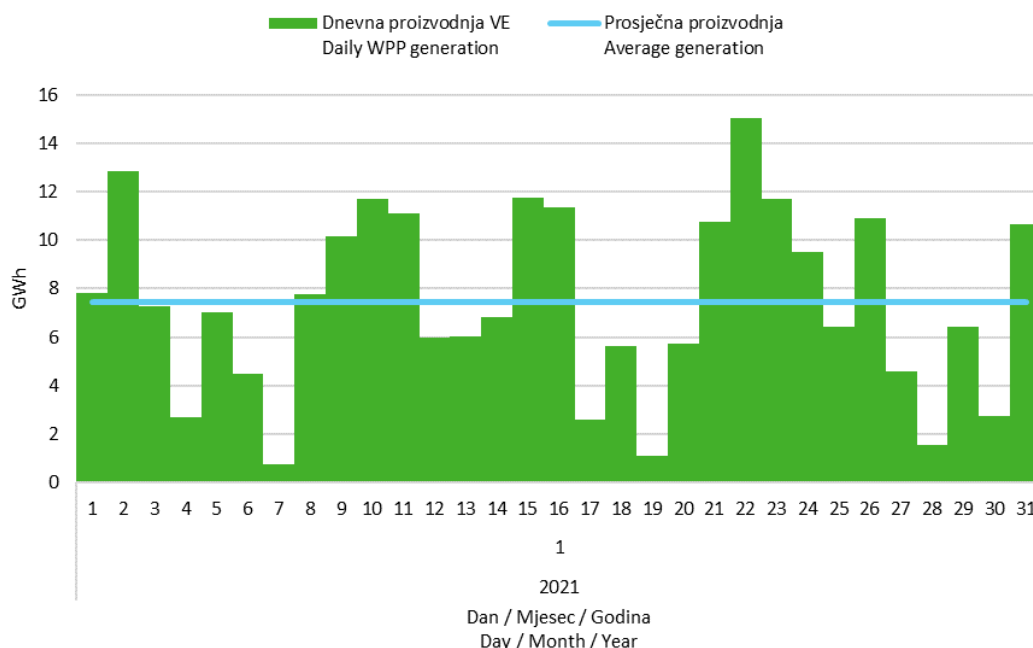
Slika 5 Dnevna proizvodnja svih vjetroelektrana u siječnju 2021. godine Figure 5 Daily generation of all wind power plants in January 2021
