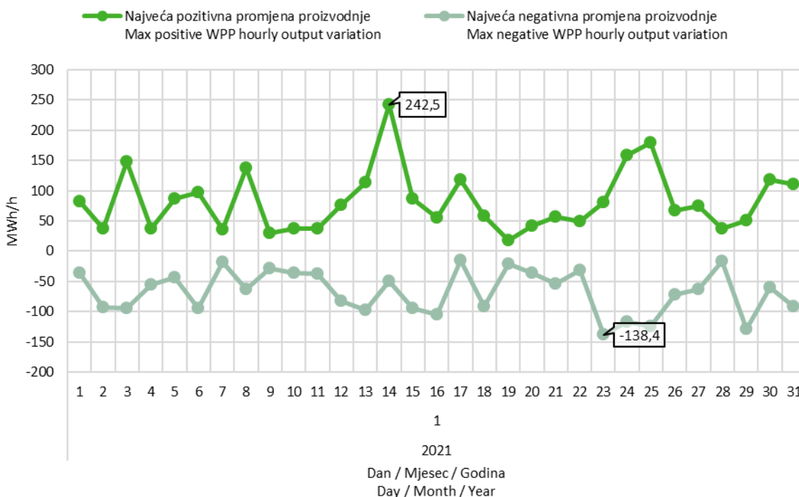
Slika 9 Maksimalna pozitivna i maksimalna negativna promjena satne proizvodnje VE u siječnju 2021. godine
