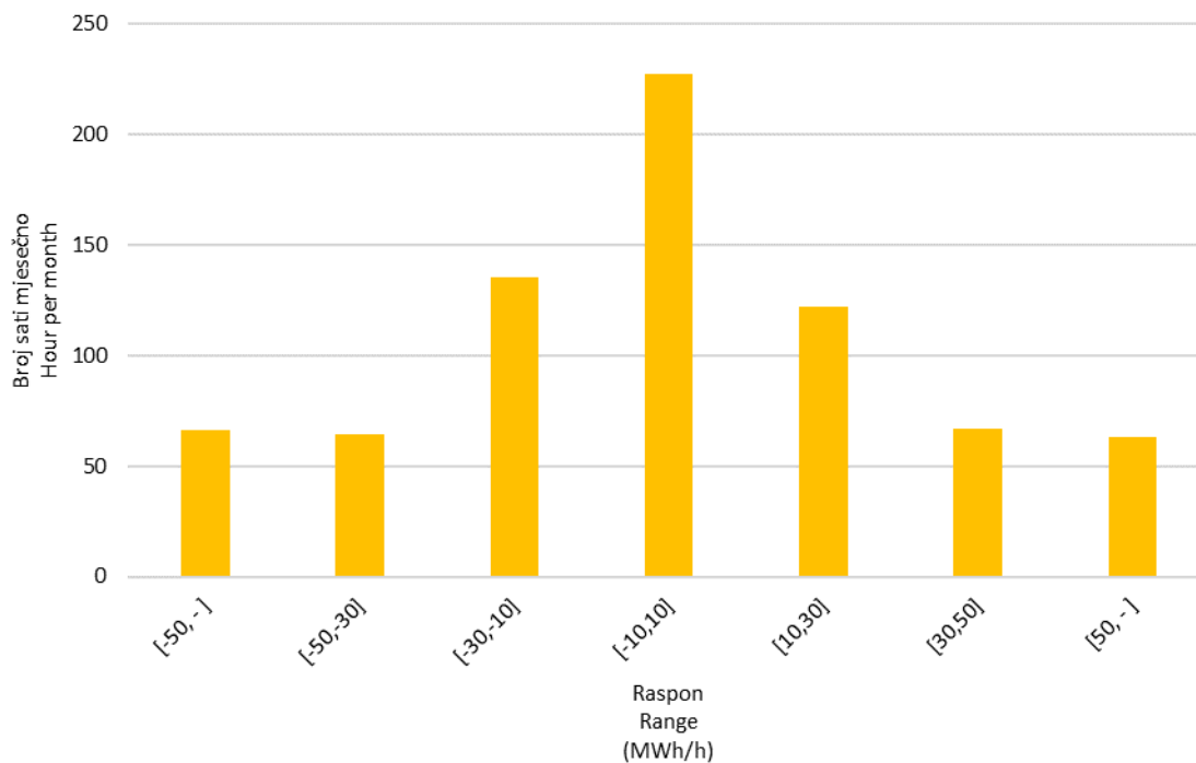
Slika 10 Statistička raspodjela satnih promjena proizvodnje VE u siječnju 2021. godine
